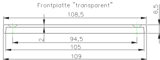
Einzelheit "A"
